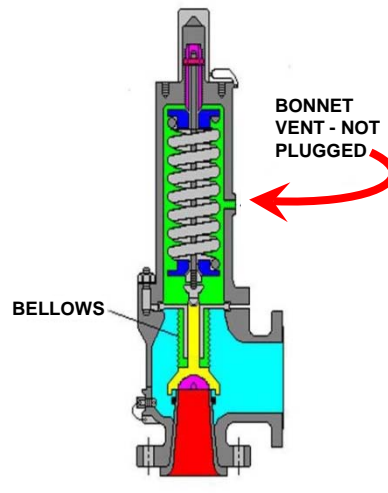
شیرهای مجهز به Balanced Bellows
