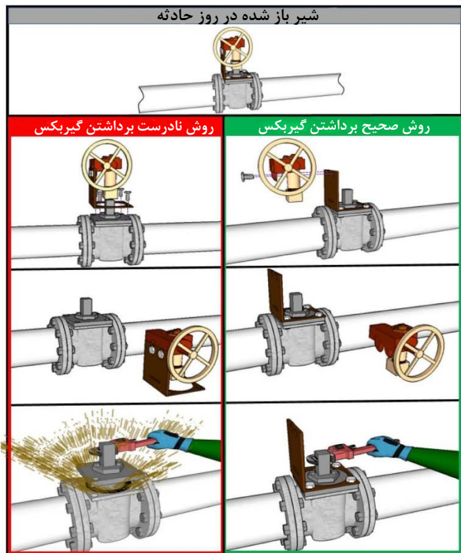
شکل ۱: نشان دادن روش صحیح و نادرست برداشتن فلکه شیر که در حادثه توضیح داده شده است (مرجع: شکل ۳ در گزارش منتشره توسط CSB به شماره 2016-02-I-LA)
