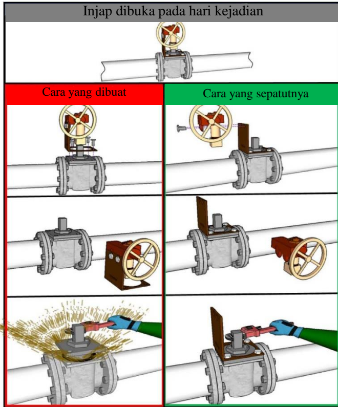
Rajah 1: Gambar rajah menunjukkan cara yang betul dan salah untuk mengeluarkan roda tangan yang diterangkan dalam kejadian (Ruj. Rajah 3 laporan CSB 2016-02-I-LA)
