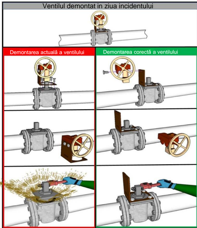
Figura 1: Diagramă arătând demontarea corectă și incorectă a roții de mână descrise în incident (Ref. Figura 3 Raportul CSB 2016-02-I-LA)
