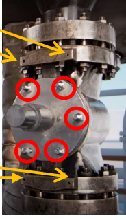
చిత్రం 2. పీడనాన్ని నిలుపుకునే వాల్వ్ కవర్ యొక్క బోల్ట్లు మరియు నట్లు హైలైట్ చేయబడ్డాయి
