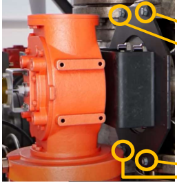
చిత్రం 1. మౌంటు బ్రాకెట్ బోల్ట్లు హైలైట్ చేయబడిన వాల్వ్ యాక్చుయేటర్
